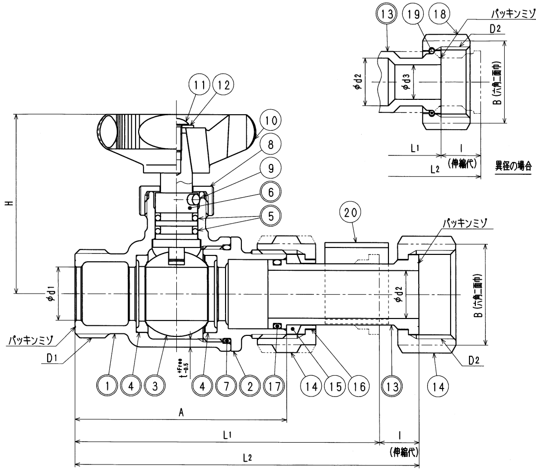
寸法表
